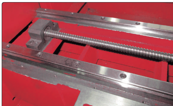
Guías lineales de ultra alta precisión
